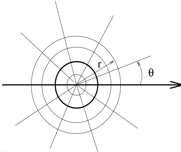
Fig. 1.1 Polar coordinates
